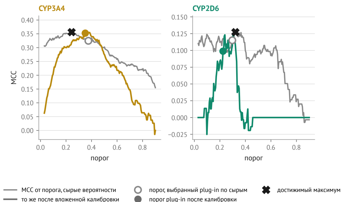
Рис. 8. MCC как функция порога. Слова «при калиброванных p_i » оказались не формальностью: на сырых вероятностях подстановочный порог промахивается мимо максимума. На CYP3A4 он даёт 0.325 при достижимых 0.358, на CYP2D6 — 0.115 при 0.127. На 3A4 промах стоит больше половины всего выигрыша от подбора порога. (Раньше в подписи стояло 0.356 против 0.358 в тексте — одна и та же величина, разошедшаяся из-за шага сетки порогов: рисунок перебирает 180 значений, f9_mccthr — 200. Точный максимум по всем различным вероятностям 0.3574.)
